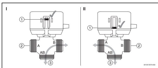
fig. 12 Caktimi i fluksit mesatar të ngrohjes
