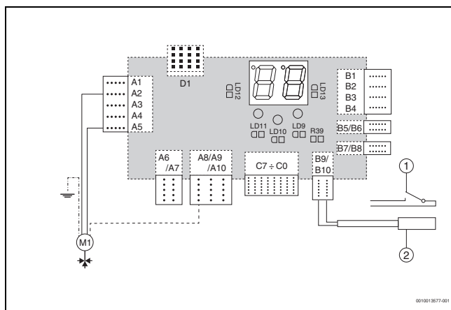
fig. 10 Lidhja e valvulës me 3 drejtime për funksionin e kontrollit të ujit të ngrohtë ose të burimit zëvendësues
