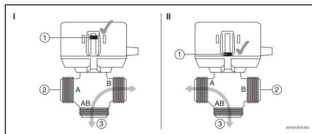
Fig. 15 Поставување на протокот на течноста за греење
