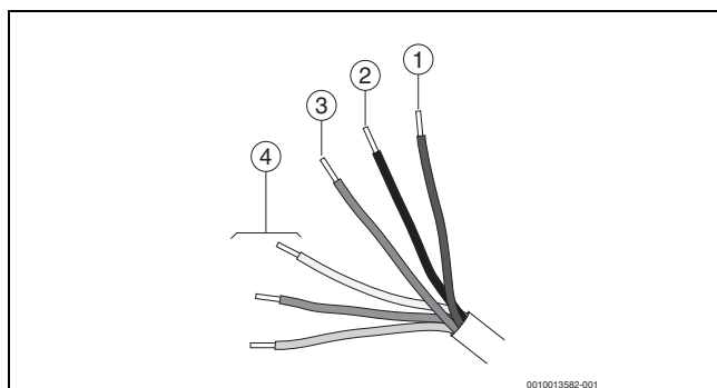
fig. 11 Lidhja e telave të aktuatorit të valvulës me 3 drejtime
