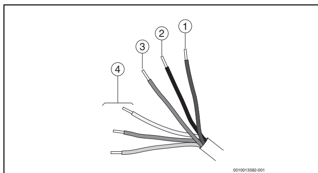
Rys. 8 Podłączanie żył elementu nastawczego zaworu 3-drogowego
