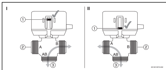
Fig. 3 Réglage du débit du fluide calorifique
