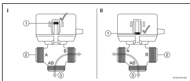
Fig. 3 Innstilling av varmemediegjennomstrømning
