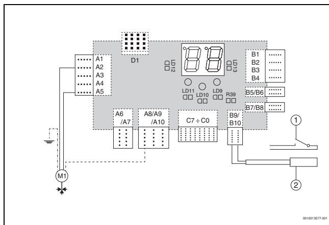
Fig. 13 Поврзување 3-насочен вентил заради контрола на топлата вода или заменскиот извор
