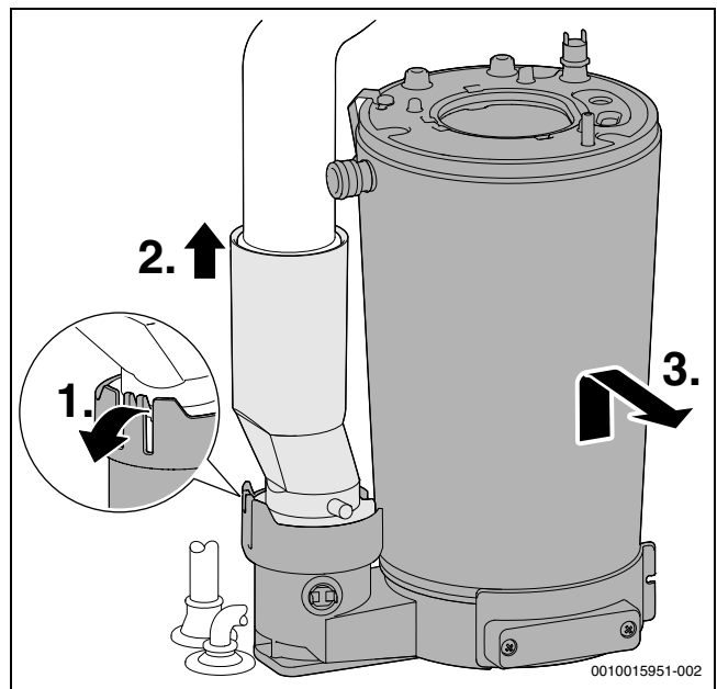
75. ábra Hőcserélő blokk kiszérése
