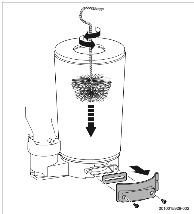
57. ábra A hőcserélő blokk tisztítása
