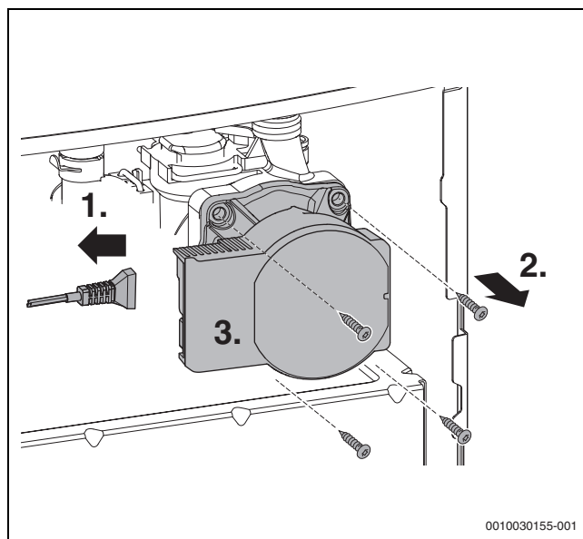
71. ábra Fűtési szivattyú kiszérése
