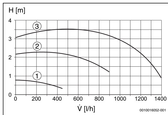
44. ábra A fűtési szivattyú jelleggörbéje (arányos nyomás)
