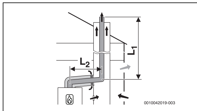
15. ábra B 53p szerinti merev füstgáz elvezetés aknában, környezeti levegőtől függő levegőellátással a felállítási helyiségben lévő koncentrikus összekötő vezetékkel keresztül; hátsó szellőzőnyílás az aknában
