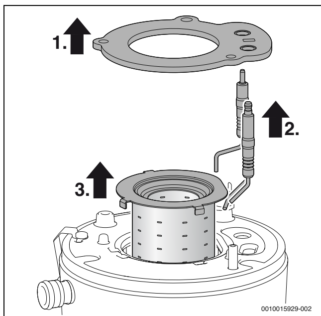
54. ábra Az égő kiszerelése
