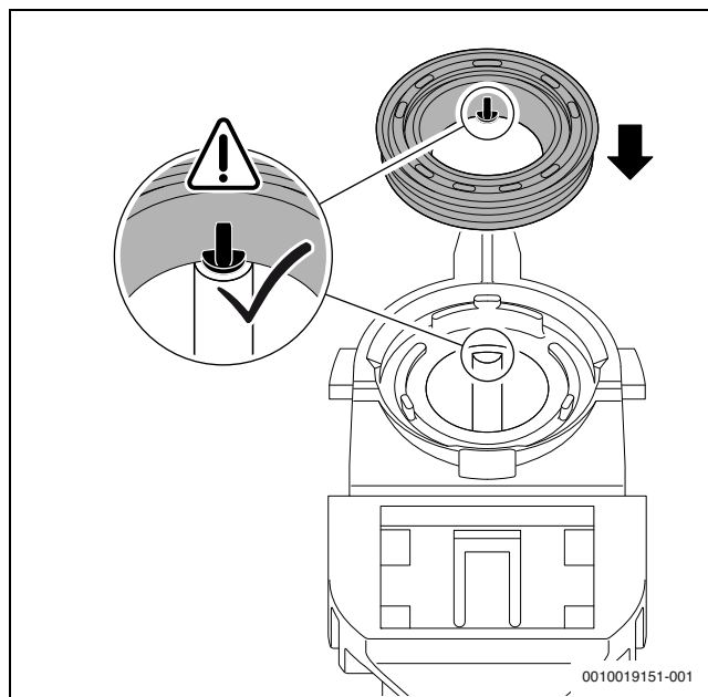
63. ábra Az új tömítés beállítása a kondenzvízszifonon
