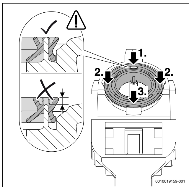
64. ábra A tömítés helyrehozása
