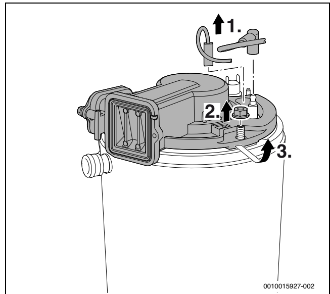
52. ábra Az égőfedél leoldása
