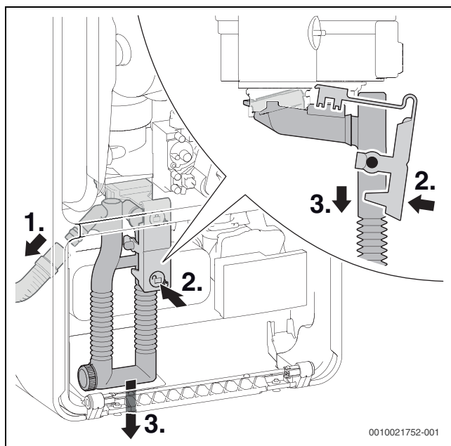
60. ábra A kondenzvíz-szifon kiserelése
