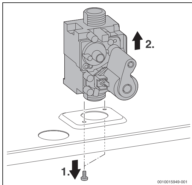
70. ábra Gázarmatúra kiszérése
