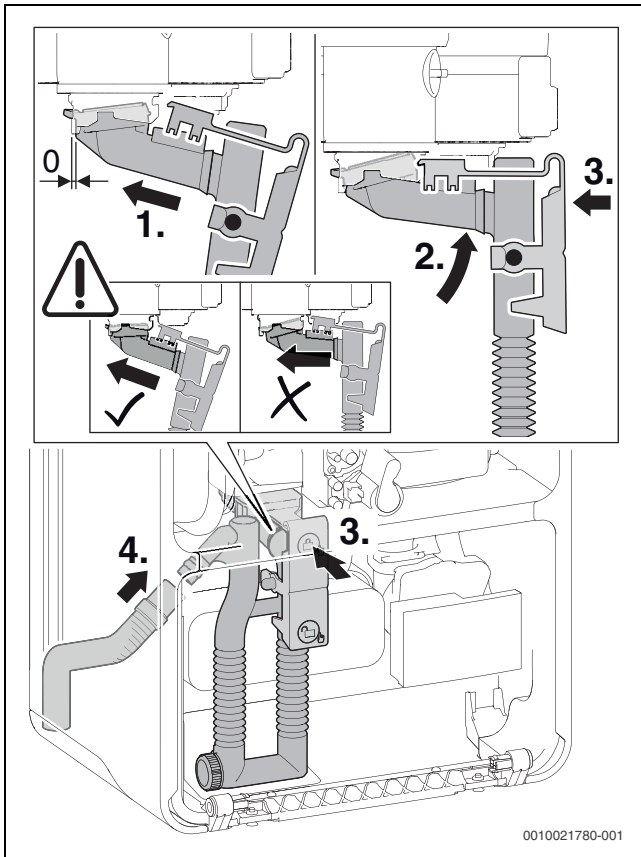
65. ábra A kondenzvízszivó behelyezése
