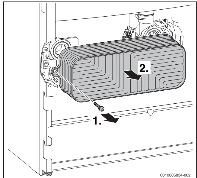
68. ábra A lemezes hőcserélő kiszérése
