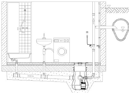
Telepítési példa - egyedüli szivattyú
