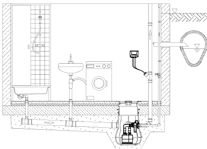
Telepítési példa - kettős szivattyú
