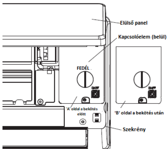
Telepítési ábra
