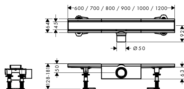
RainDrain Compact normál beépítéshez
