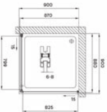
QUADRUM + QUADRUM BLACK ZUHANYKABIN
