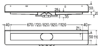
Advantix zuhanylefolyó, fal (moduláris rendszer) kombinált szigeteléshez nemesacélból, homokszórt tömítő karima Alaptest, modell 4982.20 Szagelzáró, modell 4982.92 Állítóláb-készlet, modell 4982.90 ER11 rács, matt, modell 4982.60
