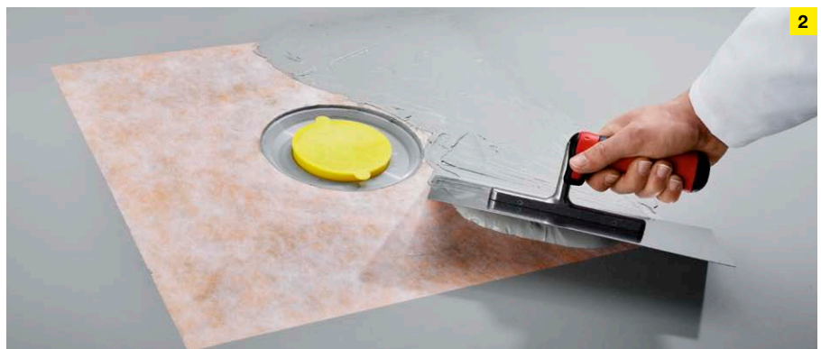
A 2. szigetelőréteg felvitele az építőipari gyakorlatban bevált kétkomponensű műanyag-cementhabarcs kombinációval.
