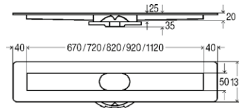
Advantix zuhanylefolyó (moduláris) kombinált szigeteléshez, nemesacélból homokszórt tömítő karima Alaptest, modell 4982.10 Szagelzáró, modell 4982.92 Állítóláb-készlet, modell 4982.90 ER10 rács, matt, modell 4982.50
