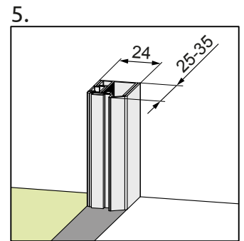
Jobbos ajtó Variant R
