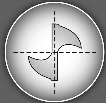
Hagyományos vágóél keresztmetszet
