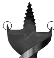
Kettős vágóélek
