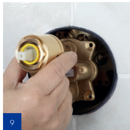
Funkciós egység beépítése
