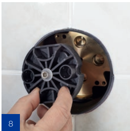
Öblítő szett egyszerű eltávolítása
