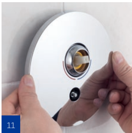
Előlap rögzítése
