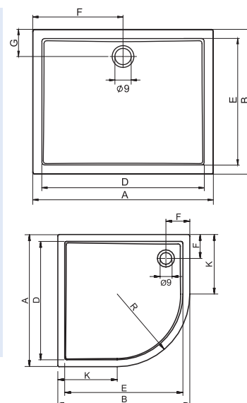
DAVOS zuhanytálcák lábbal és előlappal (magasság 14 cm):
