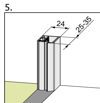
Jobbos zuhanyajtó Variant R
