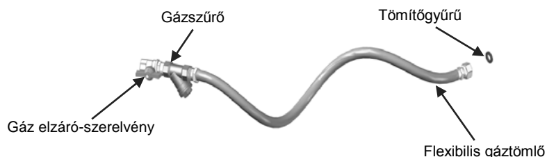
4. ábra: Csatlakoztatás flexibilis tömlővel (opció, a készülék gyártónál megvásárolható)
