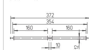
Az áttörés és rögzítés méretei mm-ben
