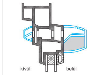
ALEF.. beépítési példa alumíniumkeretes ablakba
